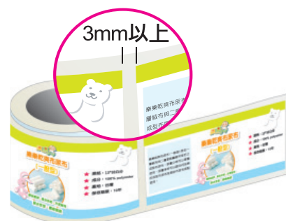
▲模與模的間距一律至少為3mm
